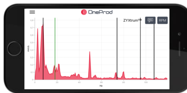
Exemplo de defeito de rolamento: uma das frequências de defeito de rolamento corresponde ao pico no ZYXtrum™
